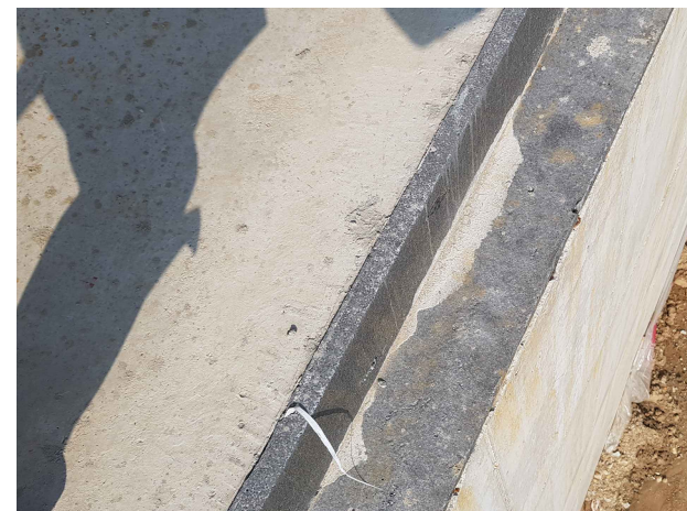
※판넬하부열교차단재설치
