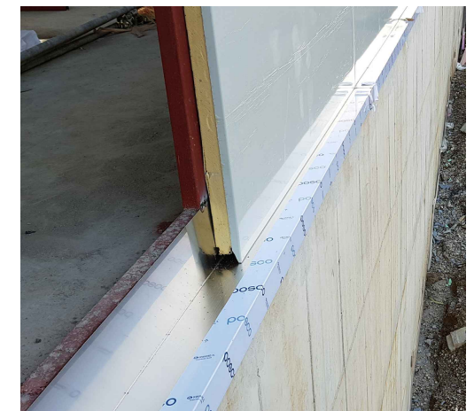
※판넬하부마감(베이스+외벽판넬)
