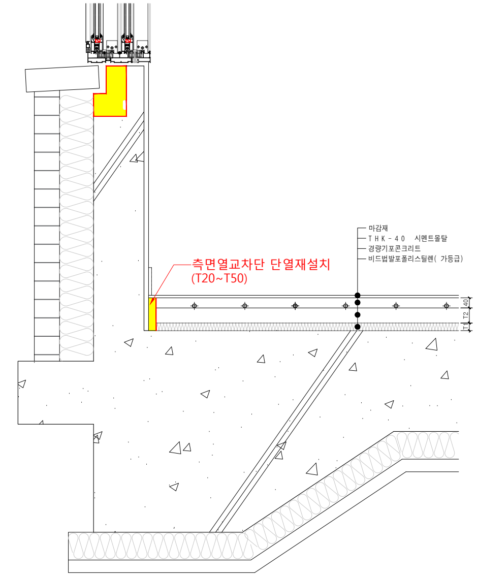
1 개선후 / 패널히팅부분 열교방지용 단열재설치 A | 02
