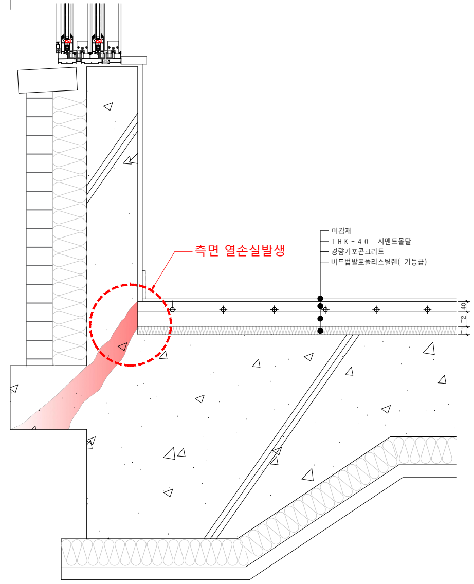
1 개선전 / 패널히팅부분 측면 열교발생 A | 01
