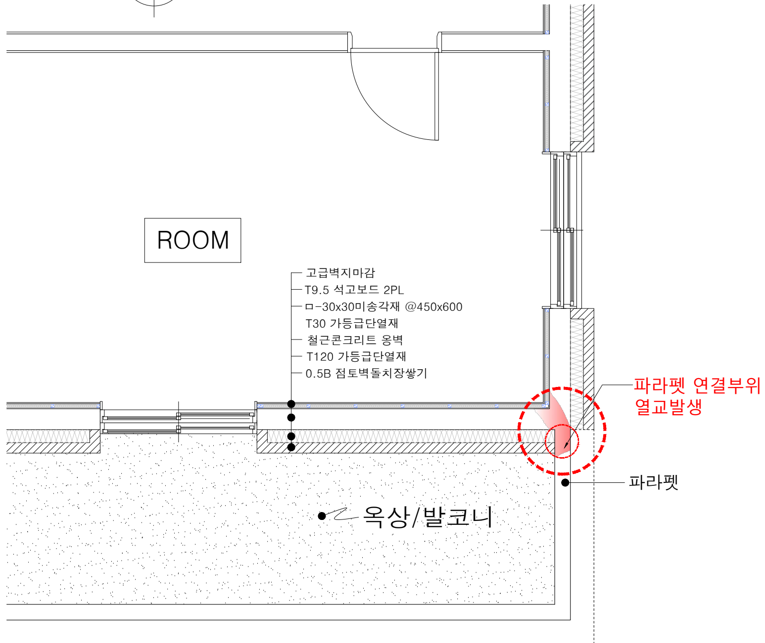
1 A 01 실내-파라펫 부분 열교발생 도면
