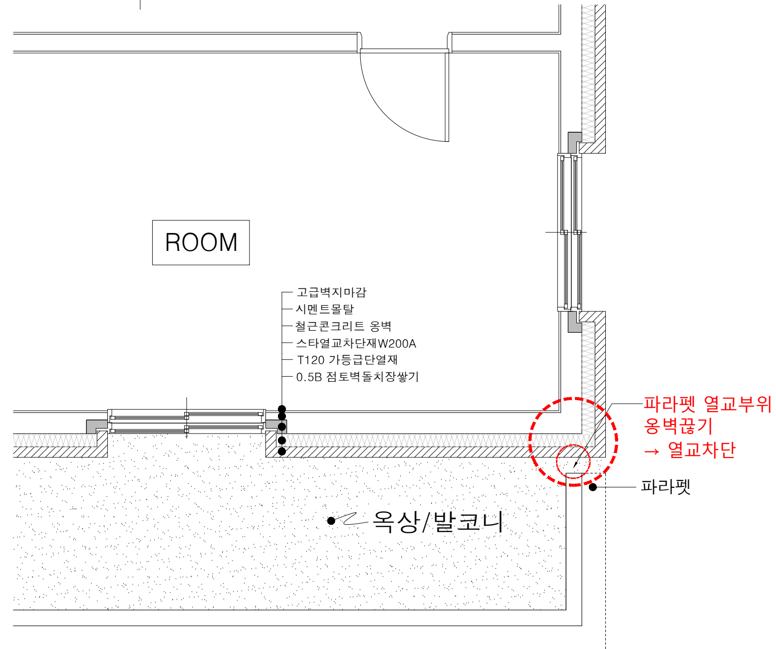
1 A 02 실내-파라펫 부분 열교차단 도면
